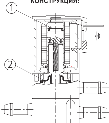
1. Катушка 2. Уплотнение
