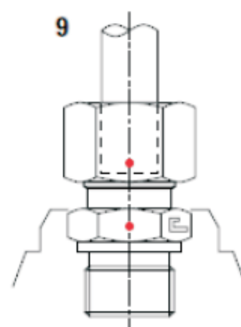
Окончательная сборка. Дозатяжка на 1/4 оборота.
