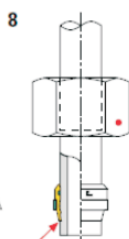
Проверка врезного кольца
