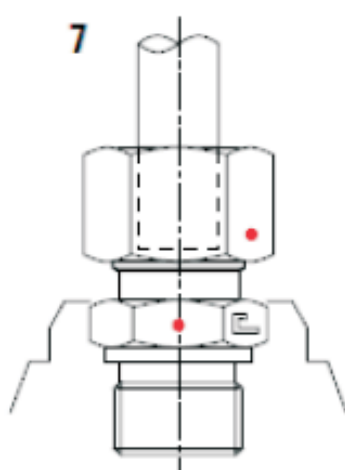
Затяжка на 3/4 оборота
