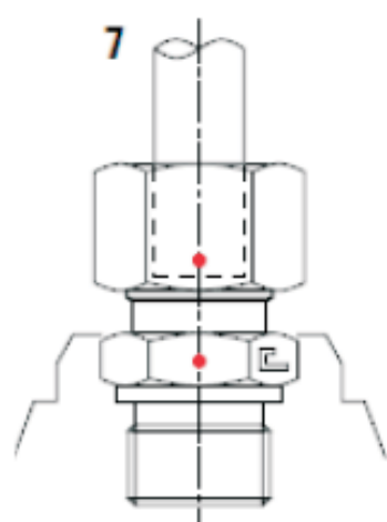
Начальная позиция предварительной сборки
