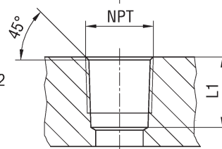
DIN 3852-2 FORM Z
