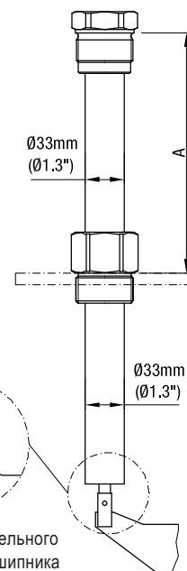
Термовставка
