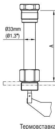
Термовставка
