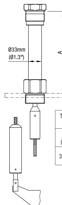
Термовставка
