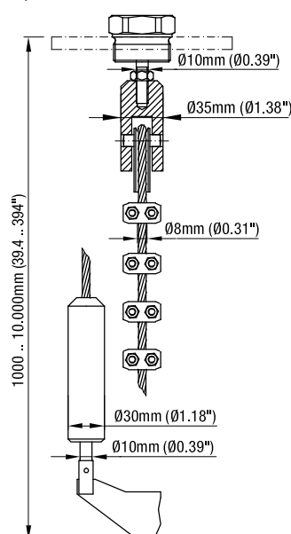
Резьба / Фланец
